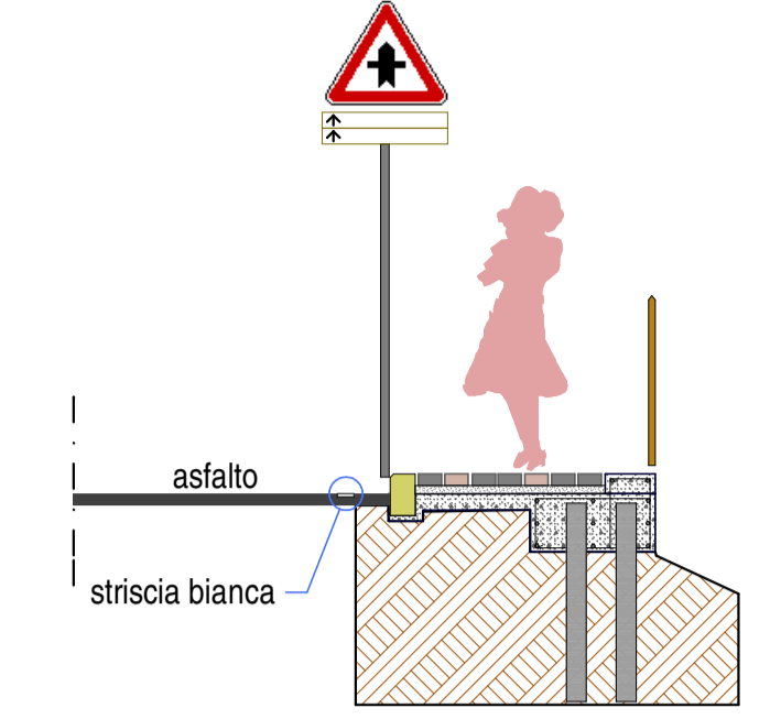
SEZIONE PROGR. 170.00
