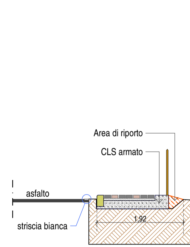
SEZIONE PROGR. 100.80
