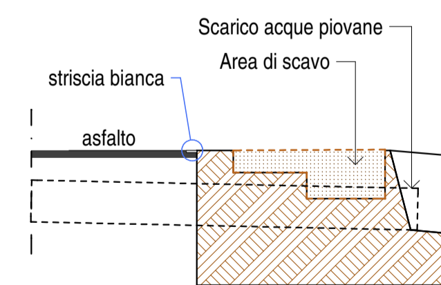
SEZIONE PROGR. 97.10
