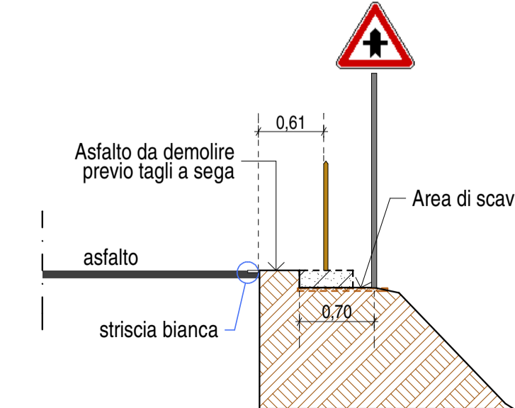
SEZIONE PROGR. 135.40
