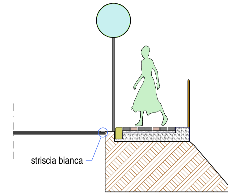
SEZIONE PROGR. 109.00
