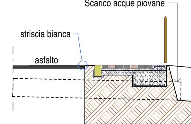
SEZIONE PROGR. 97.10
