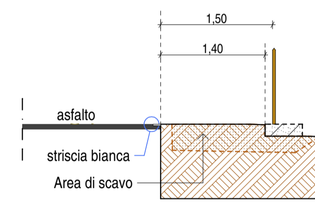
SEZIONE PROGR. 100.00
