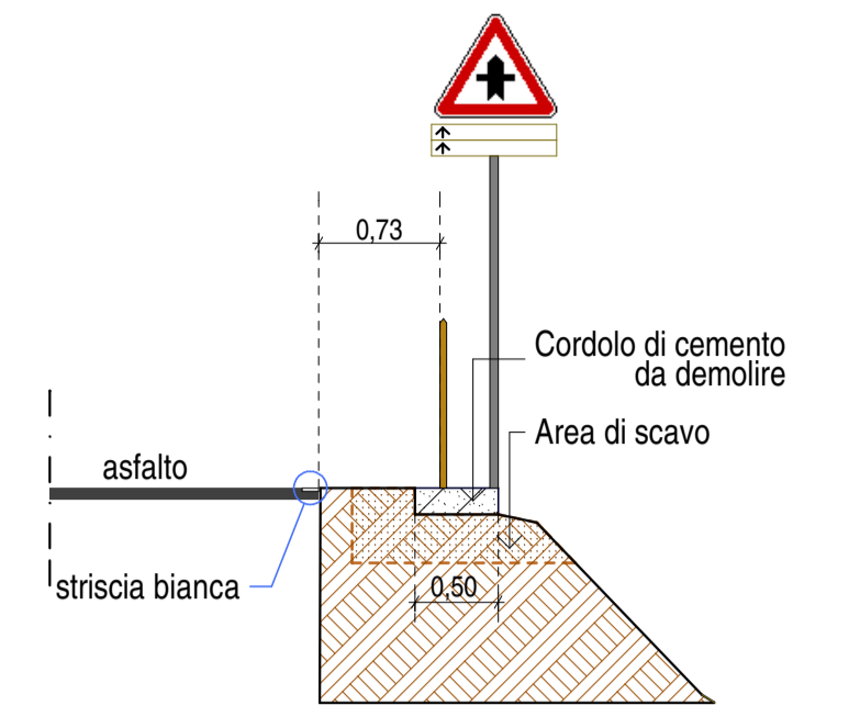
SEZIONE PROGR. 120.60
