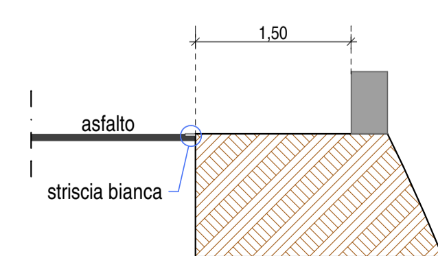
SEZIONE PROGR. 95.00
