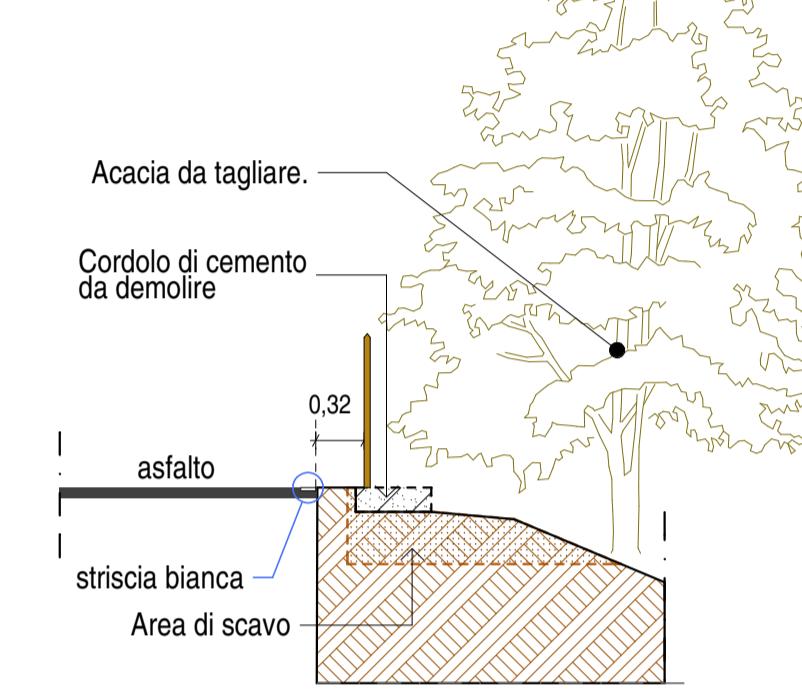
SEZIONE PROGR. 152.90
