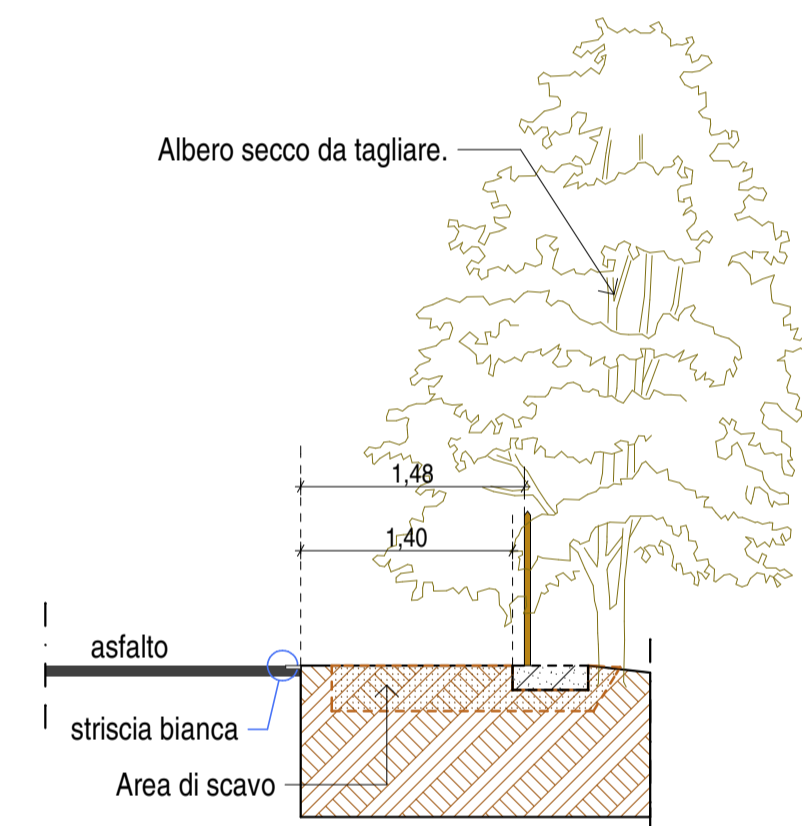
SEZIONE PROGR. 100.80
