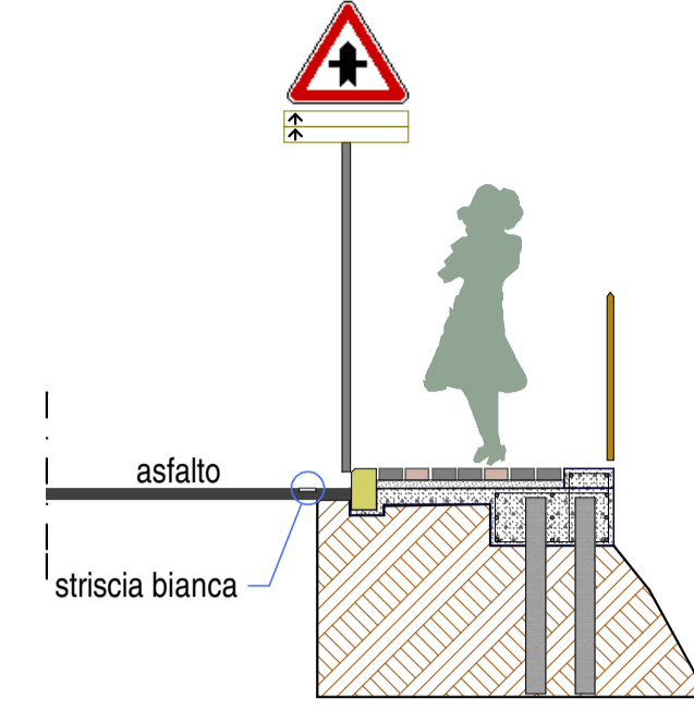
SEZIONE PROGR. 120.60
