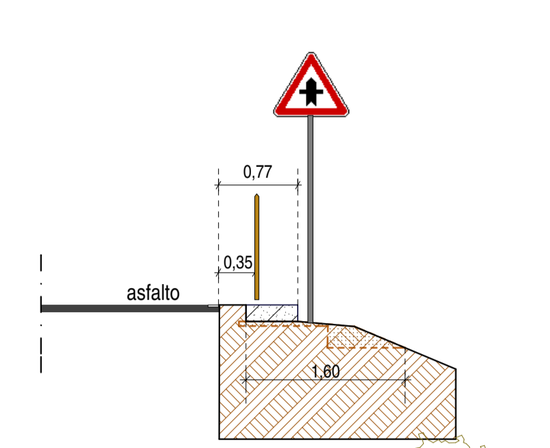
SEZIONE PROGR. 170.00
