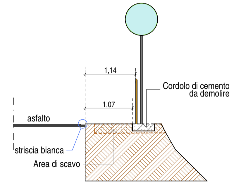
SEZIONE PROGR. 109.00
