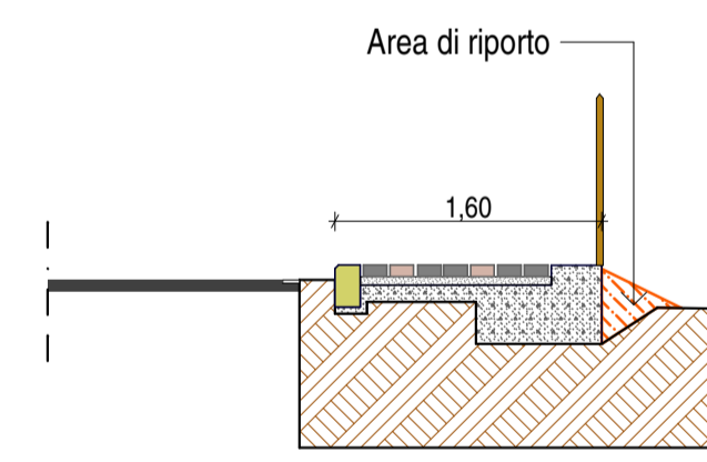
SEZIONE PROGR. 100.00
