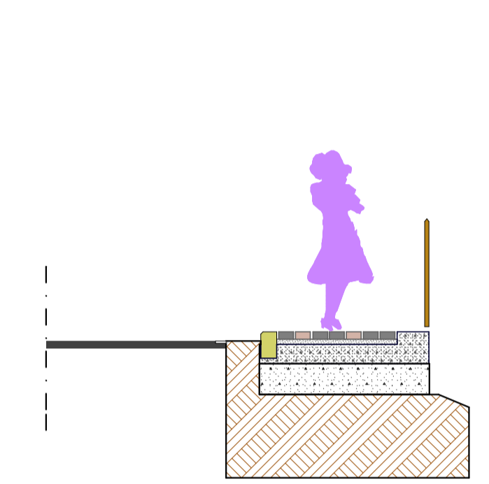
SEZIONE PROGR. 152.90
