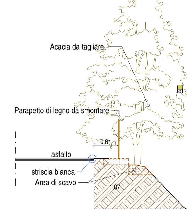
SEZIONE PROGR. 140.40
