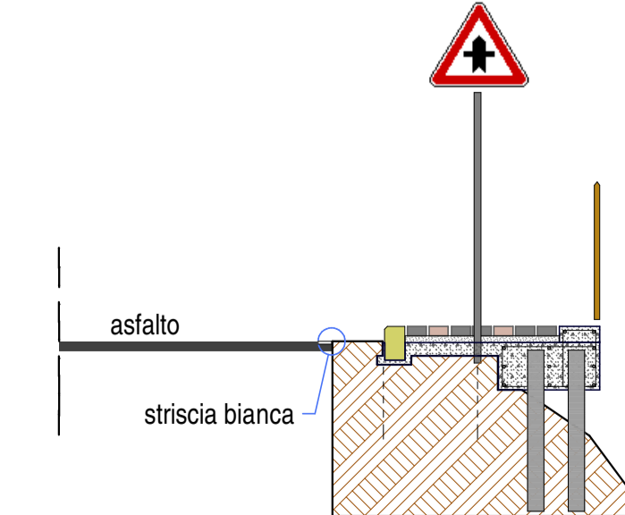
SEZIONE PROGR. 135.40
