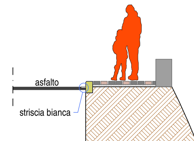
SEZIONE PROGR. 95.00
